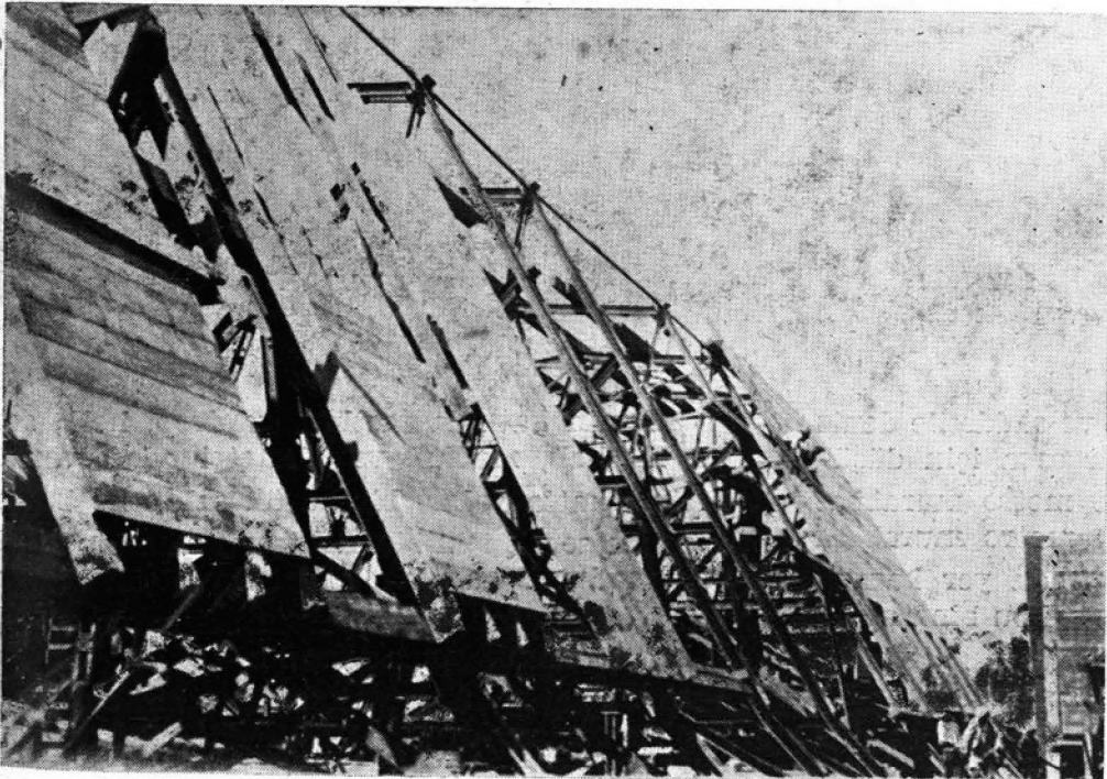
Haydarpaşa garı çatısı — Muhtelif inşaat safhaları.
